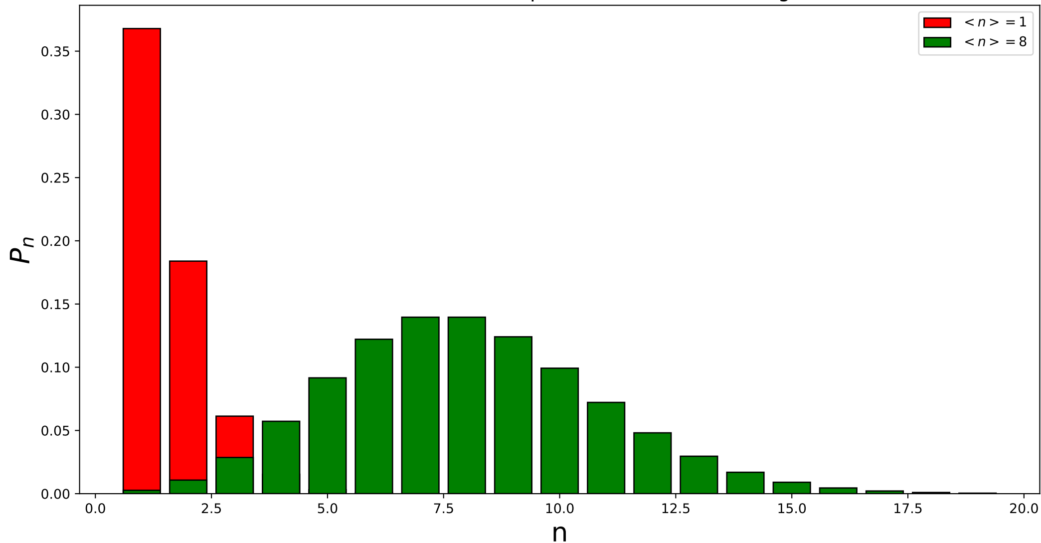
Distribución de Poisson para los cuantos de energía n
